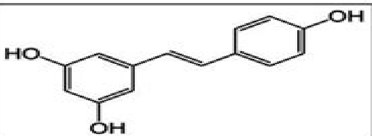
Stilbenes
